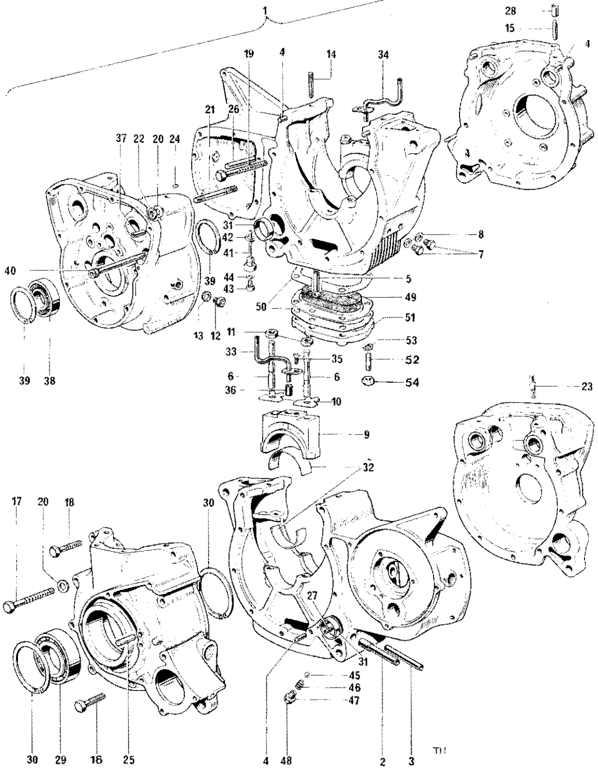
Fig. 2. CRANKCASES
