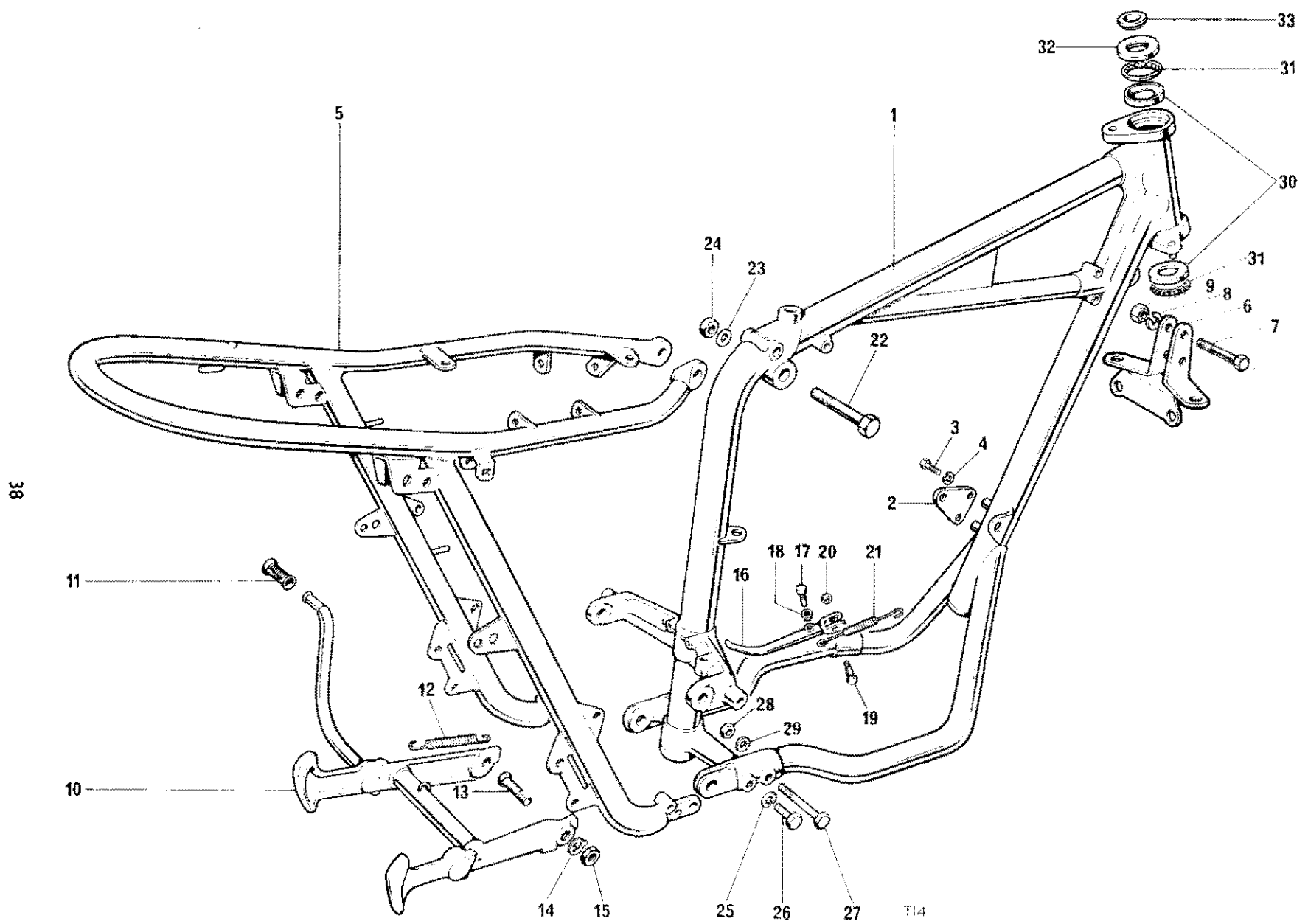
Fig. 16. FRAME
