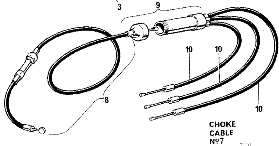
Fig. 31. CONTROL CABLES
