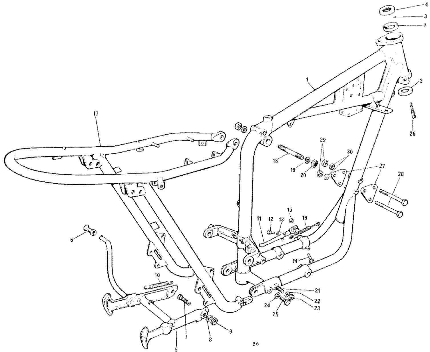
Fig. 12. FRAME
