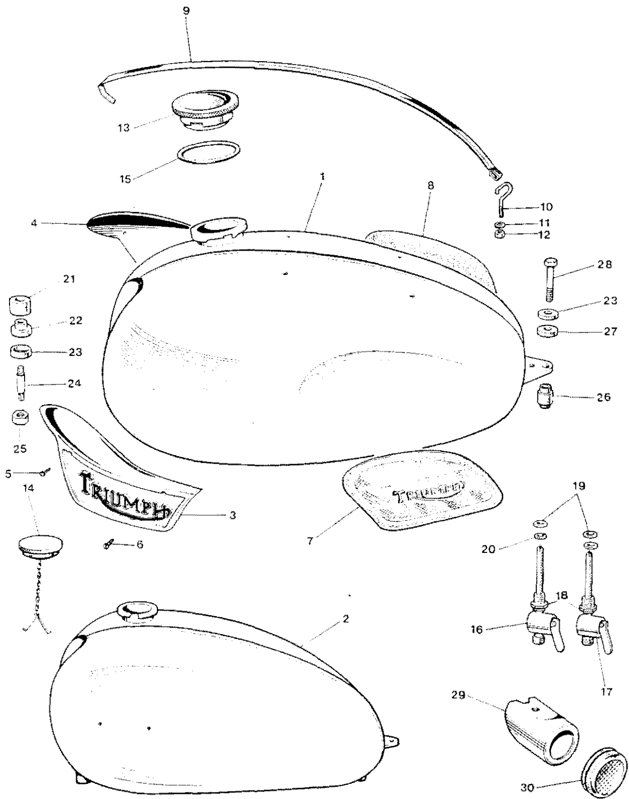
Fig. 21. GAS TANKS
