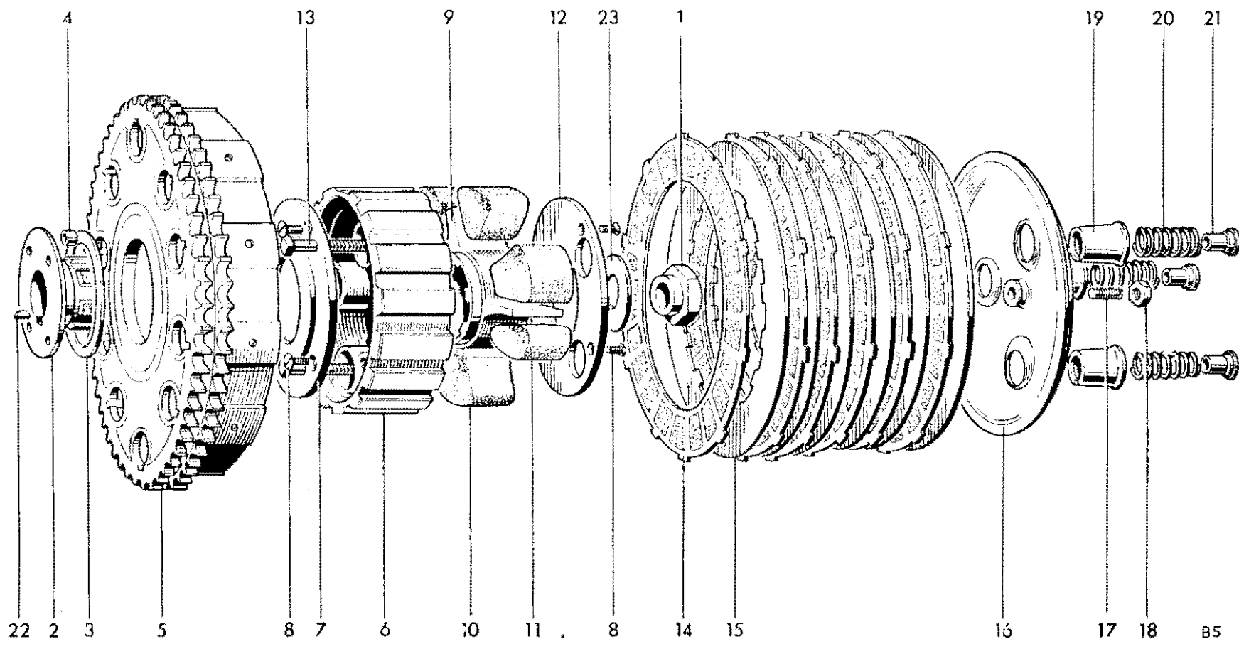
Fig. 10. CLUTCH
